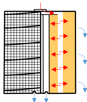
Konštrukcia typu SW-42
