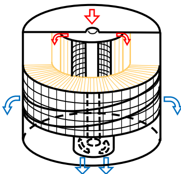
Konštrukcia typu SW-42
