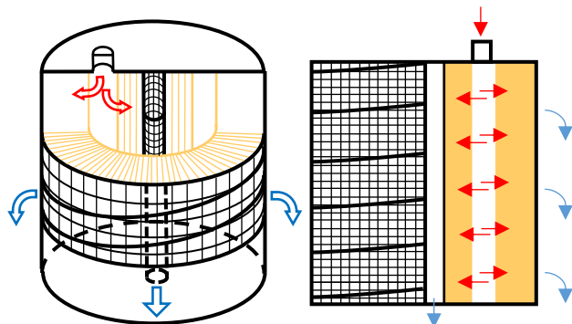
Klasická konštrukcia
