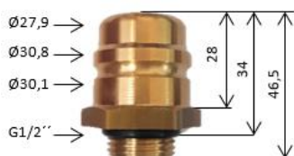
Typ A – G1/2\"
