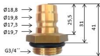
Typ B – G3/4\"
